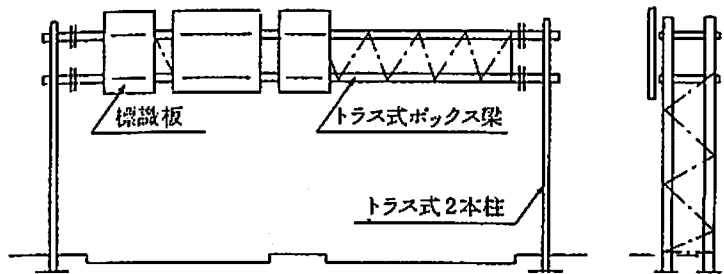
オーバ－ヘッド(トラス型)
